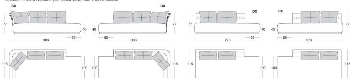
Penisola / Peninsula / Диван с приставным элементом / Угловой элемент
