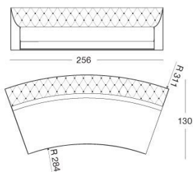
Centrale tondo / Round central / Центральные секции круглый
