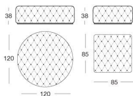
Centrale tondo / Round central / Центральные секции круглый
