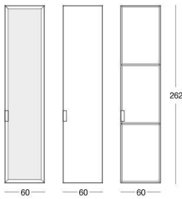
Ante per modulo 60 cm e angolare Doors for 60 cm and corner modules Створки для модуля 60 см и углового модуля
