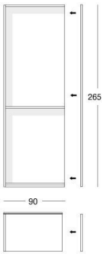
Modulo 90 cm / Module 90 cm / Модуль 90 см
