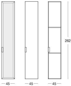
Ante per modulo 90 cm Doors for module 90 cm Створки для модуля 90 см
