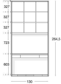
Spaziature ripiani / Shelf spacing / Проставки между полками
