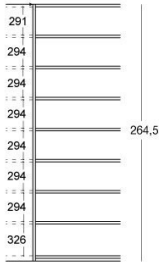
Spaziature ripiani / Shelf spacing / Проставки между полками
