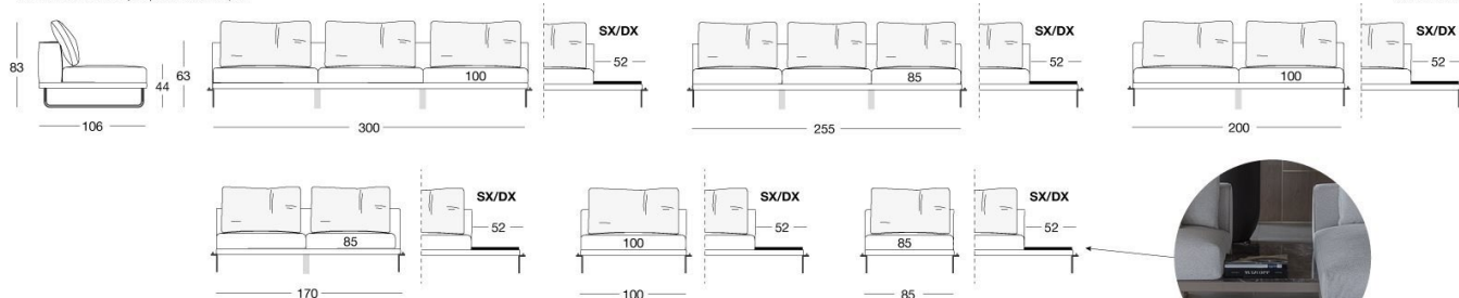
Centrali / Central / Центральные секции
